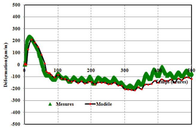
Figure 1 : Confrontation des prédictions du modèle aux mesures de la corde vibrante CV3
