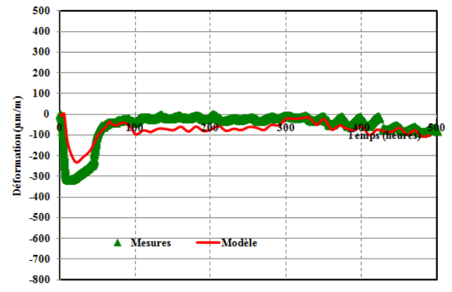
Figure 1 : Confrontation des prédictions du modèle aux mesures de la jauge électrique SUP1
