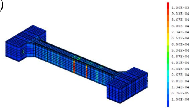
Figure 1 : Faciès de fissuration à la fin de l'essai THM du bloc RG9 : à gauche : relevé visuel in situ et à droite : modélisation
