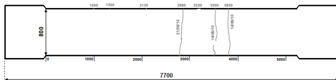
Figure 1 : Faciès de fissuration à la fin de l'essai THM du bloc RG9 : à gauche : relevé visuel in situ et à droite : modélisation
